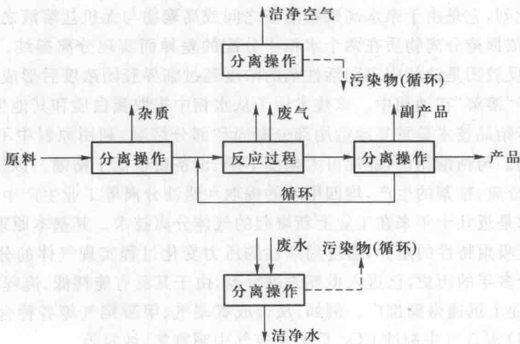
图 1-1 生产过程中的分离操作
