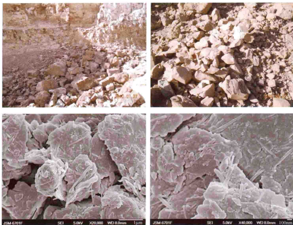
图 1-31 靖远凹凸棒石黏土矿及其 SEM 图片
