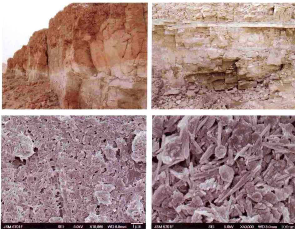
图 1-29 临泽正北山凹凸棒石黏土矿及其 SEM 图片
