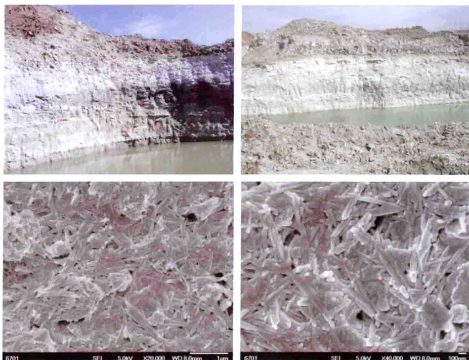
图 1-23 黄泥山凹凸棒石黏土矿及其 SEM 图片
