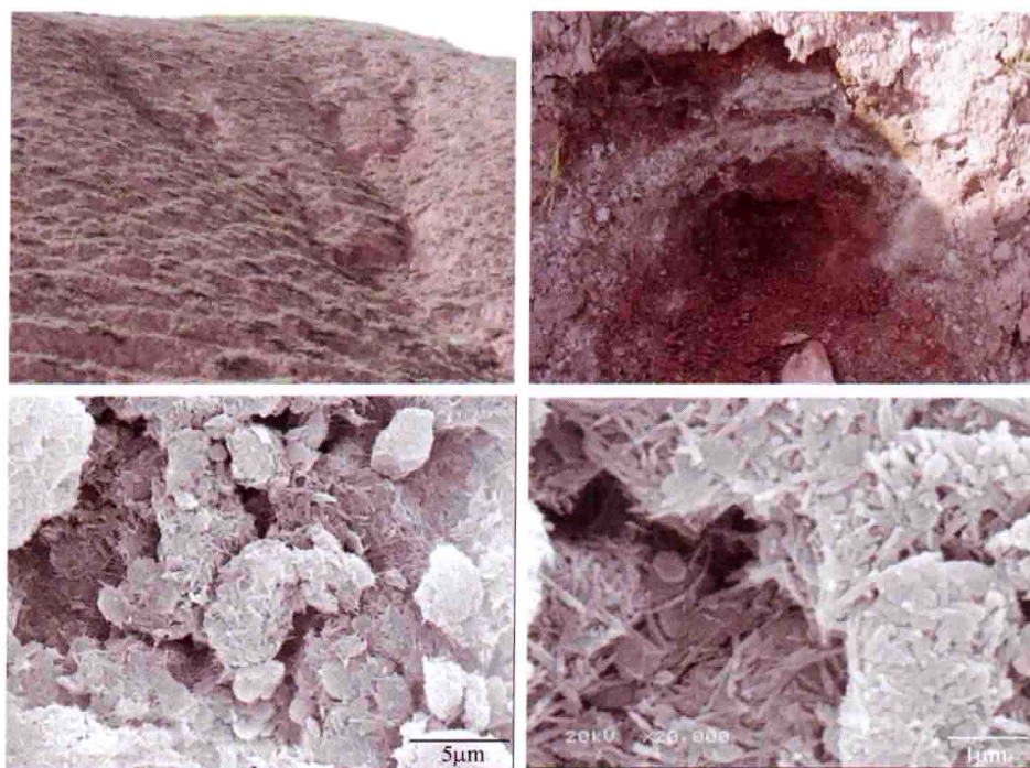
图 1-30 会宁凹凸棒石黏土矿及其 SEM 图片
