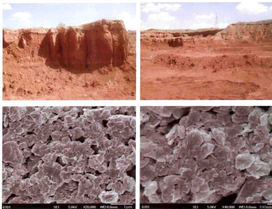
图 1-36 巴拉贡矿区和黏土矿物的 SEM 图片
