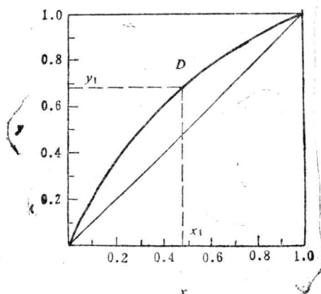
图1-2 苯—甲苯混合液的 x - y 图
