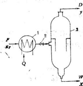
图1-7 平衡蒸馏装置
