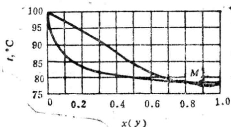
图1-3 常压下乙醇—水溶液的 t-x-y 图
