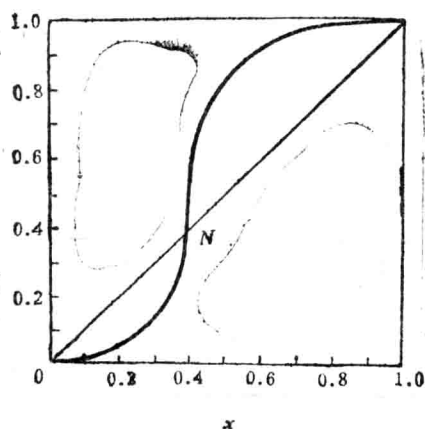
图1-6 常压下硝酸—水溶液的 x-y 图
