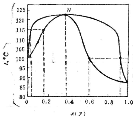
图1-5 常压下硝酸—水溶液的 t-x-y 图
