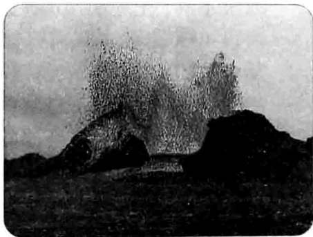
火山喷发
