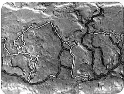
海底地图（深色粗线条为板块分界线）
