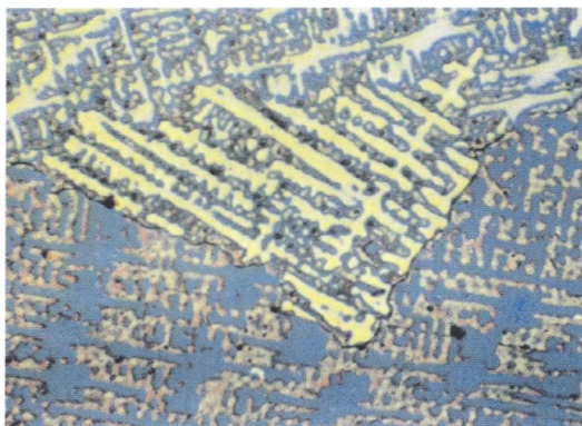
彩图3 冷模铸造的5% Sn青铜 150×
