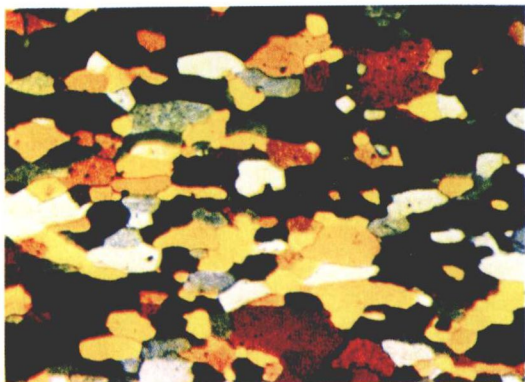
彩图 1 试样经电解抛光并阳极复膜(偏光)100×
