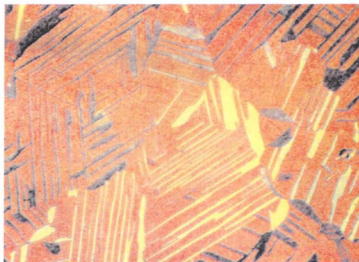
彩图4 热染后的钛-铝化合物为基的合金 100×
