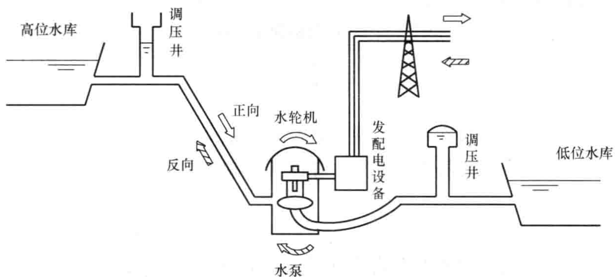
图 0-2 水力发电厂与抽水蓄能电厂示意图
