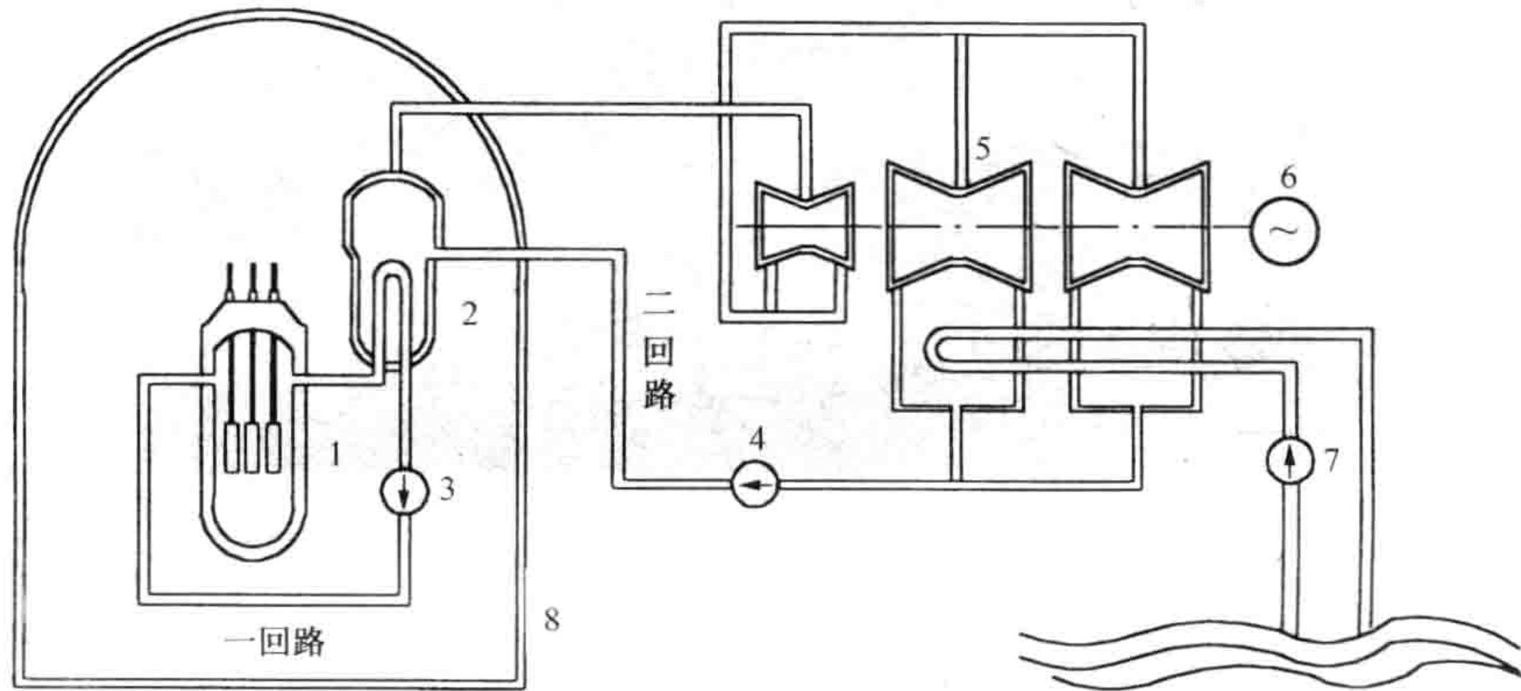
图 0-4 核电站简要流程图
