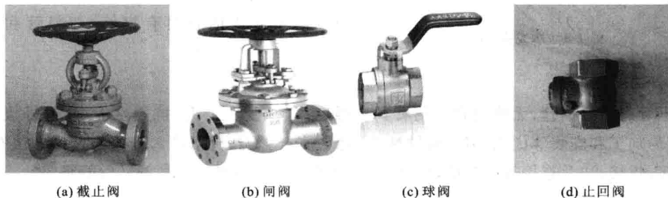
图 1-6 阀门
