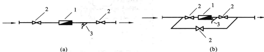
图 1-4 水表节点
