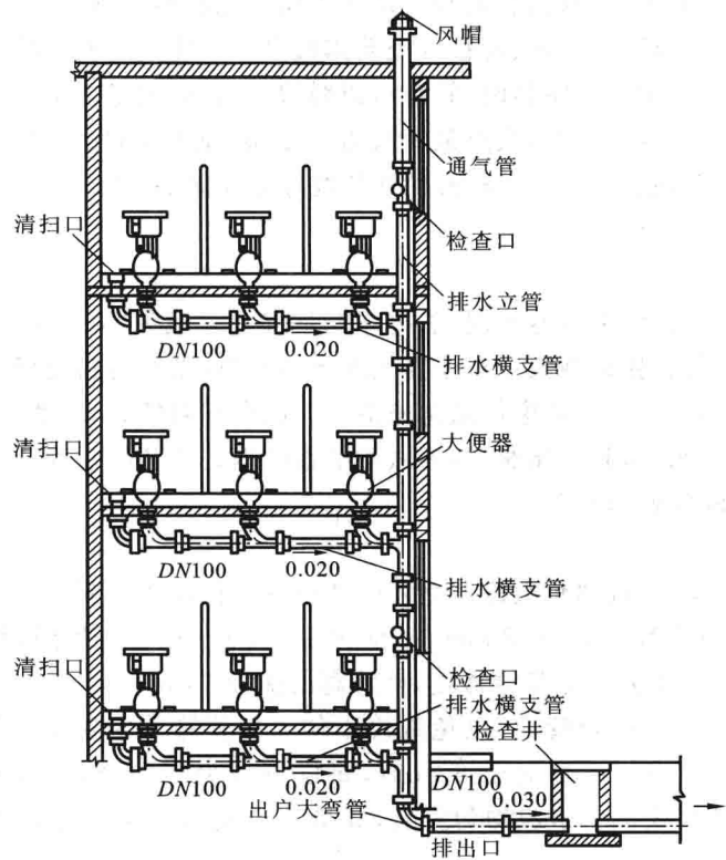
图 1-12 建筑内部生活污水排水系统
