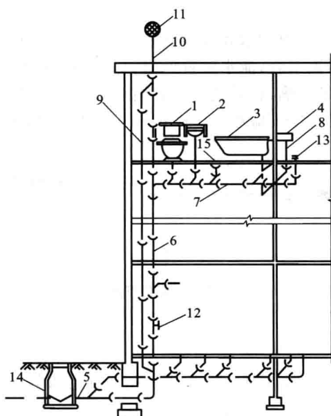
图 1-3 排水系统图
