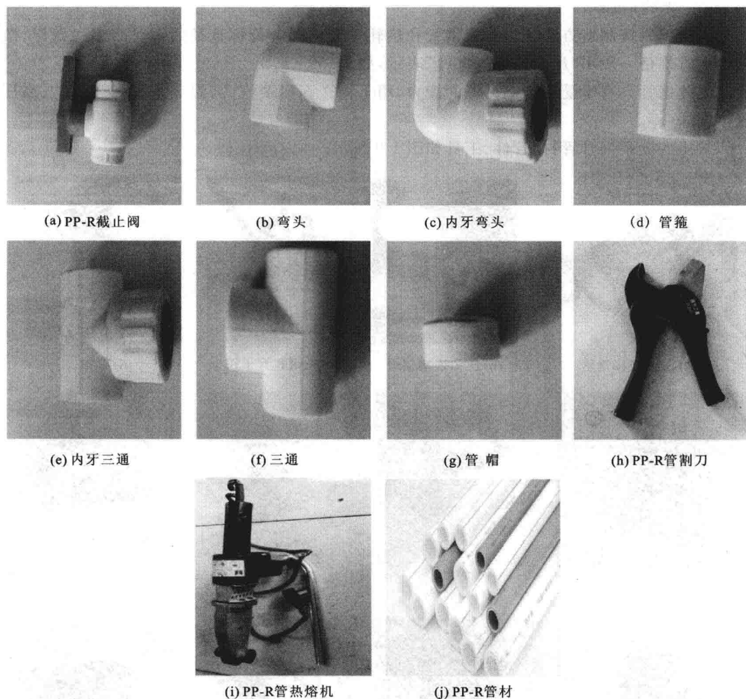
图 1-10 PP-R 管、管件和热熔工具
