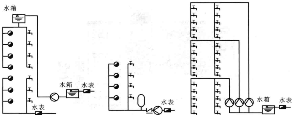
图 1-2 给水系统图
