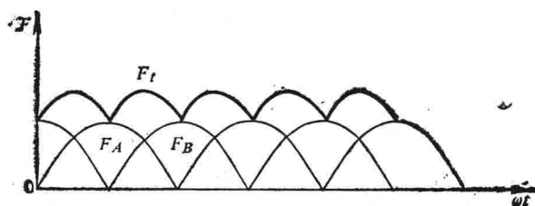
图1-6 电磁吸力曲线
