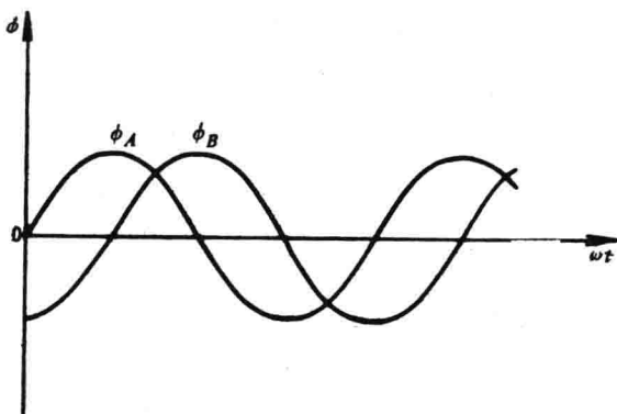
图1-5 磁通曲线
