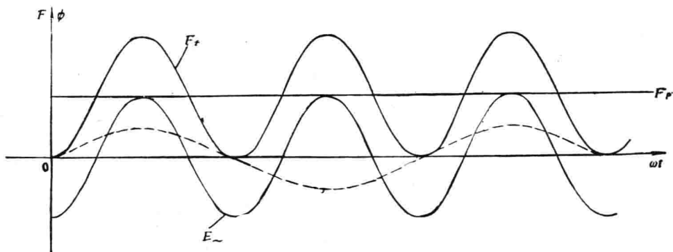
图1-3 吸力、磁通随时间变化的曲线
