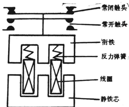
图1-2 电磁式交流接触器原理图
