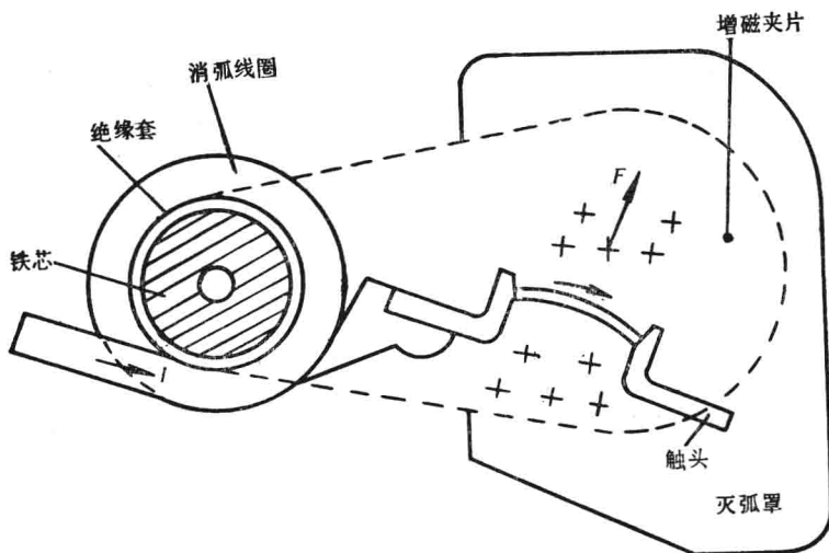
图1-9 磁吹装置
