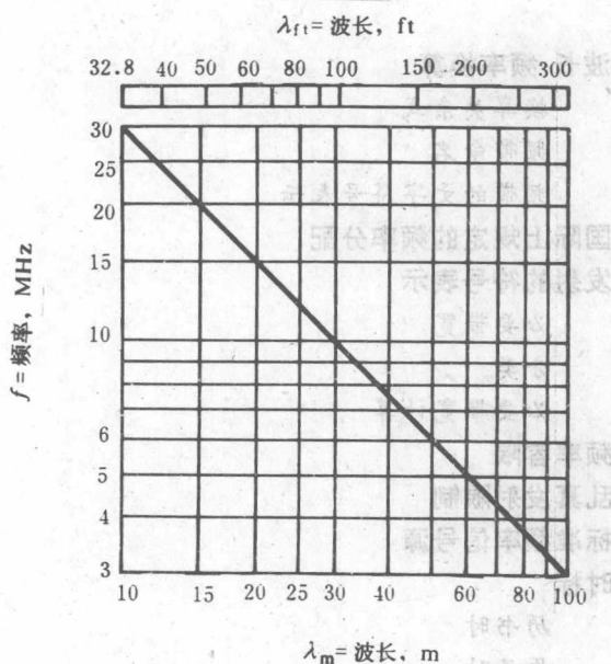
图 1. 波长-频率换算
