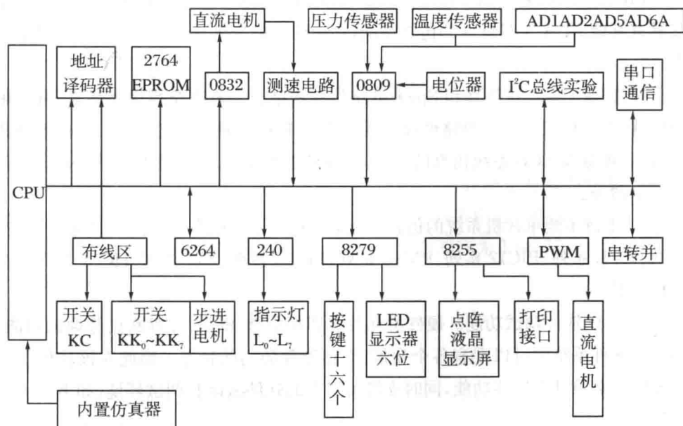
图 1.1 ZY11201D 实验箱逻辑模块结构图
