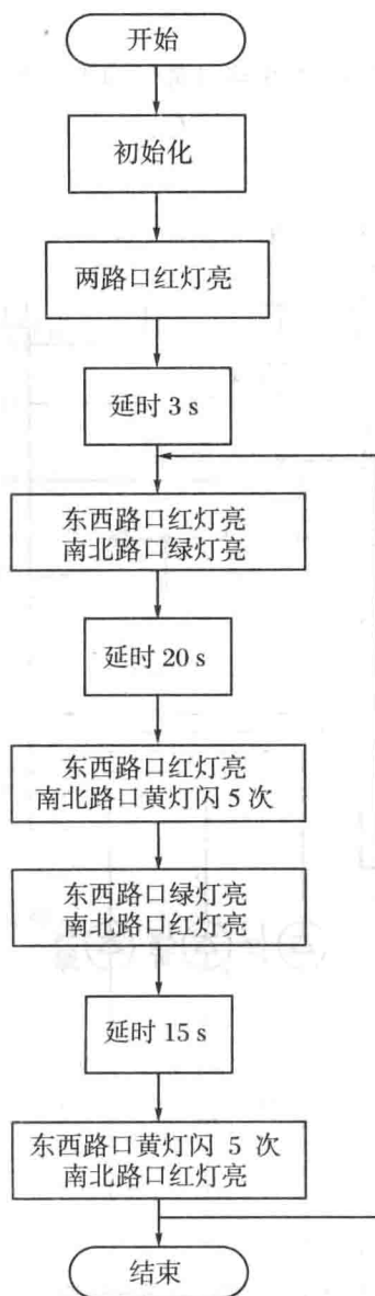
图 1.5 实验二流程图
