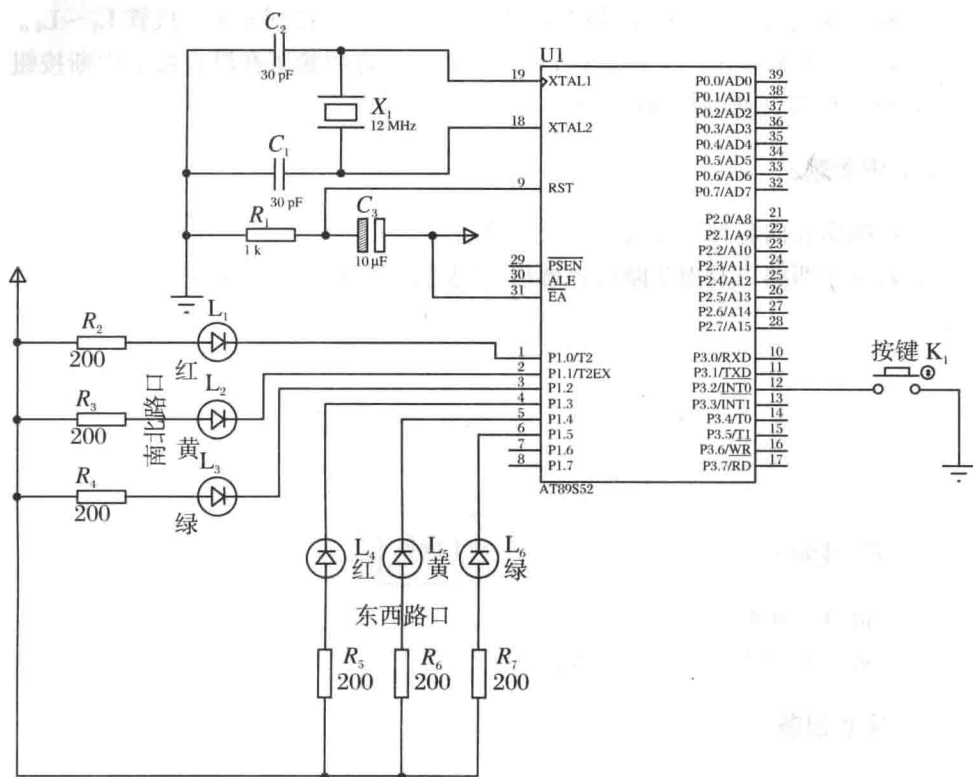
图 1.6 实验三电路原理图
