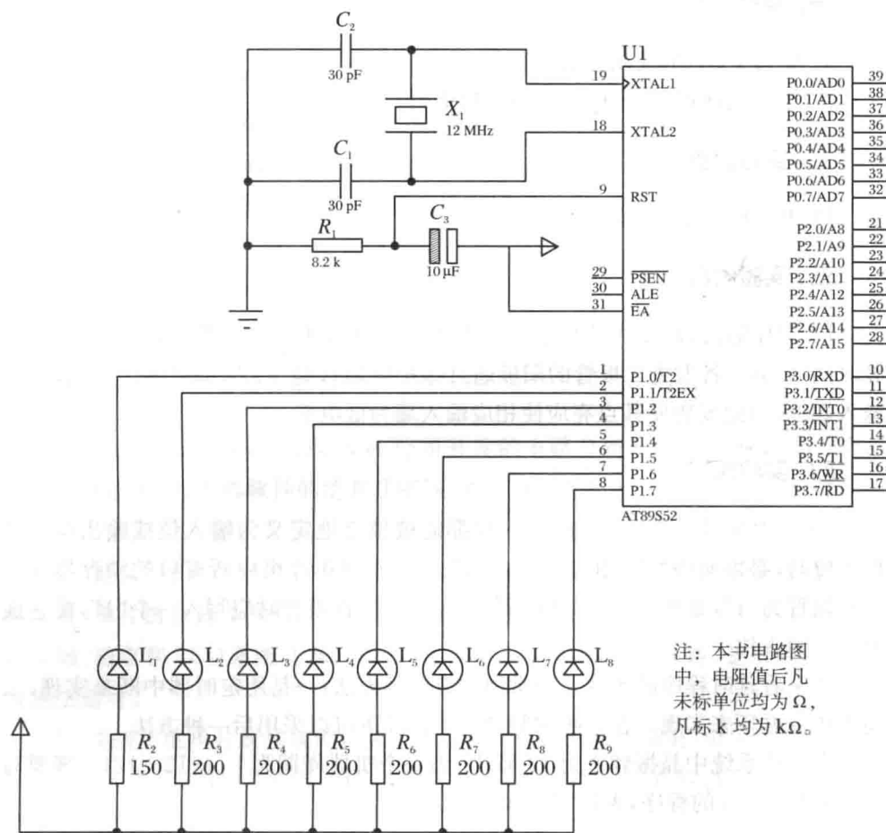
图 1.2 实验一电路原理图
