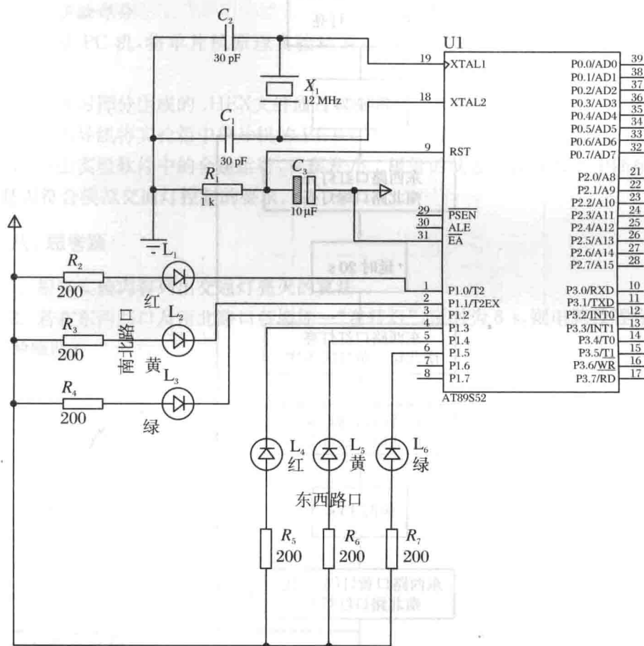
图 1.4 实验二电路原理图
