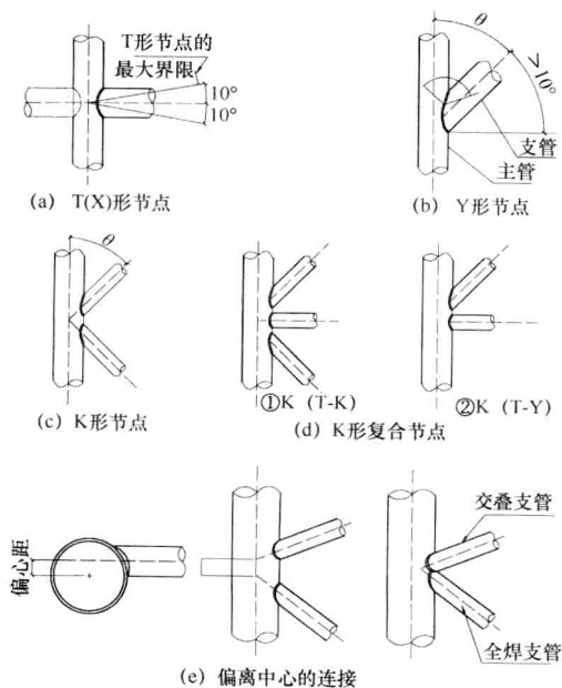
图 5.2.1 管结构节点形式
