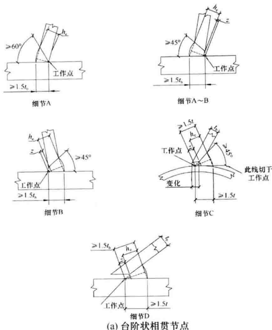
图 5.3.6-4 管材相贯节点部分焊透焊缝各区坡口形式与尺寸 (一)
