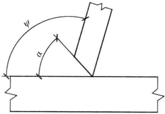
图 5.3.6-2 局部两面角 \Psi 和坡口角度 \alpha
