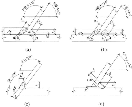
图 5.3.4 斜角角焊缝计算厚度
