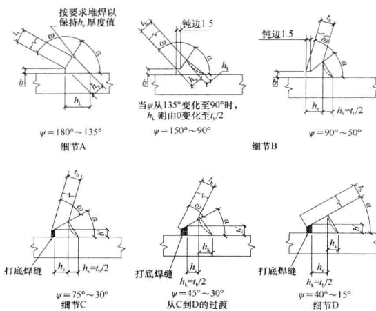
图 5.3.6-3 管材相贯节点全焊透焊缝的各区域坡口形式与尺寸(焊缝为标准平直状剖面形状)
