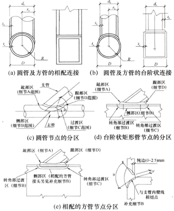
图 5.3.6-1 圆管、矩形管相贯节点焊缝分区
