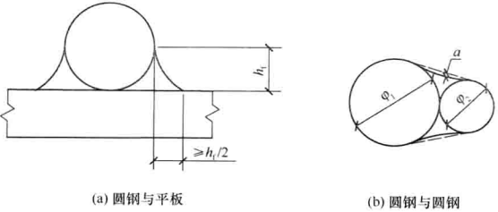
图 5.3.5 圆钢与平板、圆钢与圆钢焊缝计算厚度 式中： \varphi_1 ——大圆钢直径，mm； \varphi_2 ——小圆钢直径，mm； a ——焊缝表面至两个圆钢公切线的间距，mm。
