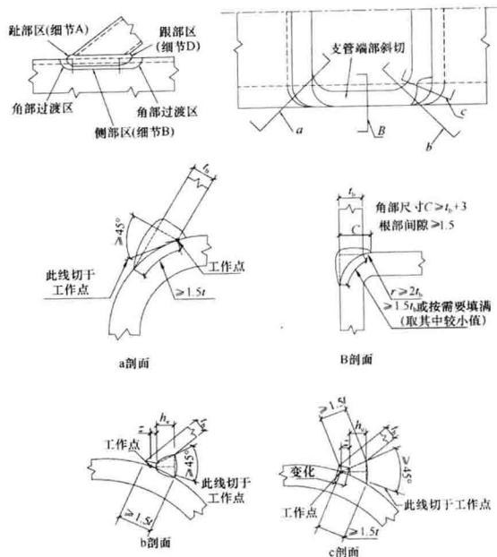
图 5.3.6-4 管材相贯节点部分焊透焊缝各区坡口形式与尺寸 (二)
