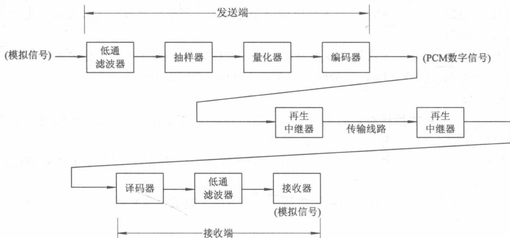
图 2-1 脉冲编码调制(PCM)的模型
