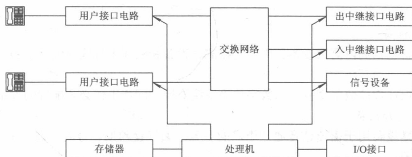
图 1-6 程控数字交换机的组成框图
