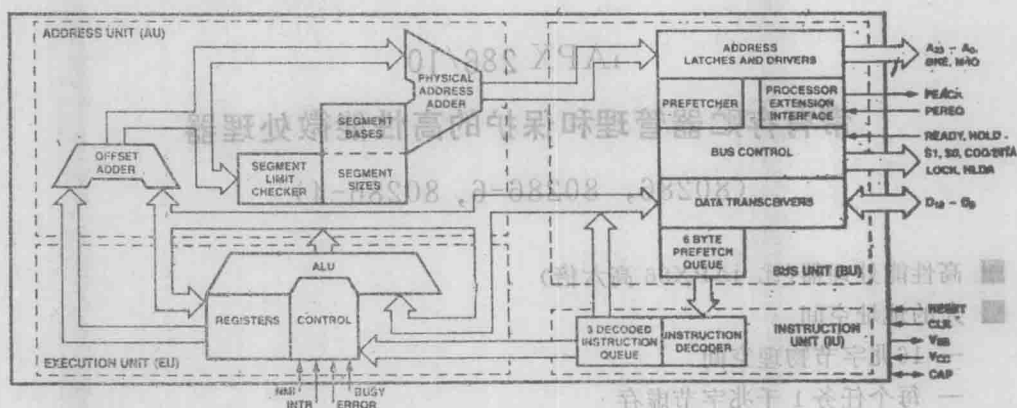
图 1 80286内部框图
