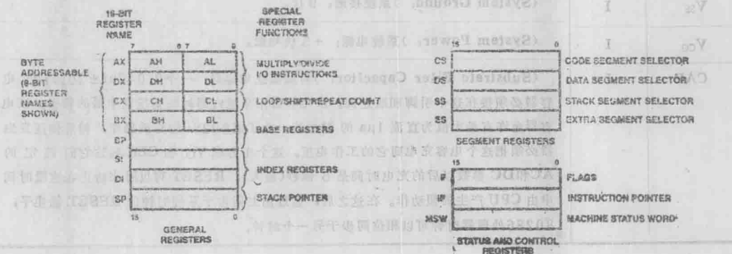
图 3 寄存器集
