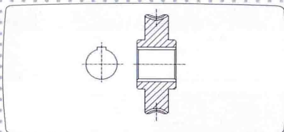
蜗轮
