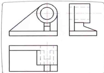
绘制轴承座
