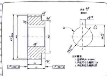
直齿圆柱齿轮
