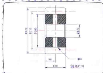
油泵齿轮
