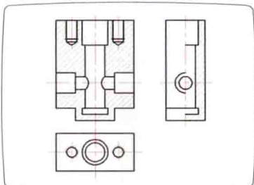
绘制阀体
