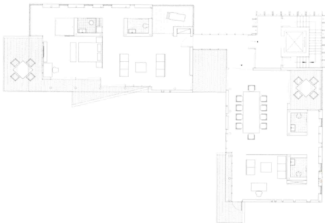
3F Plan/三层平面图
