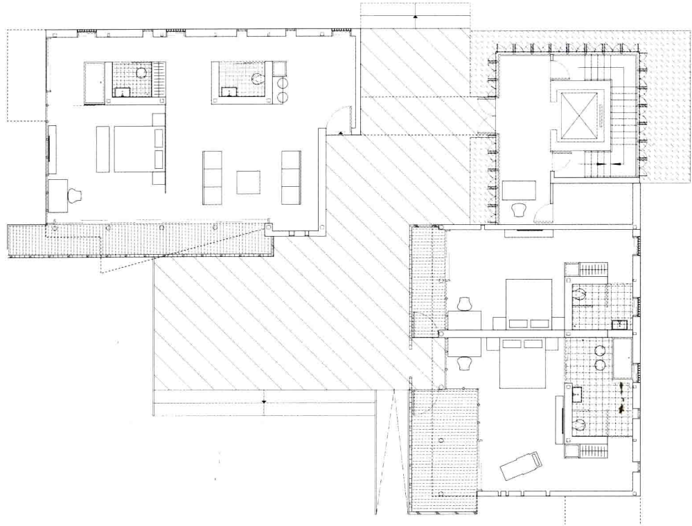
1F Plan/一层平面图
