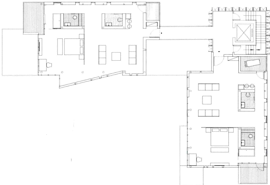
2F Plan/二层平面图
