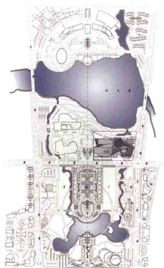
区域总平面
