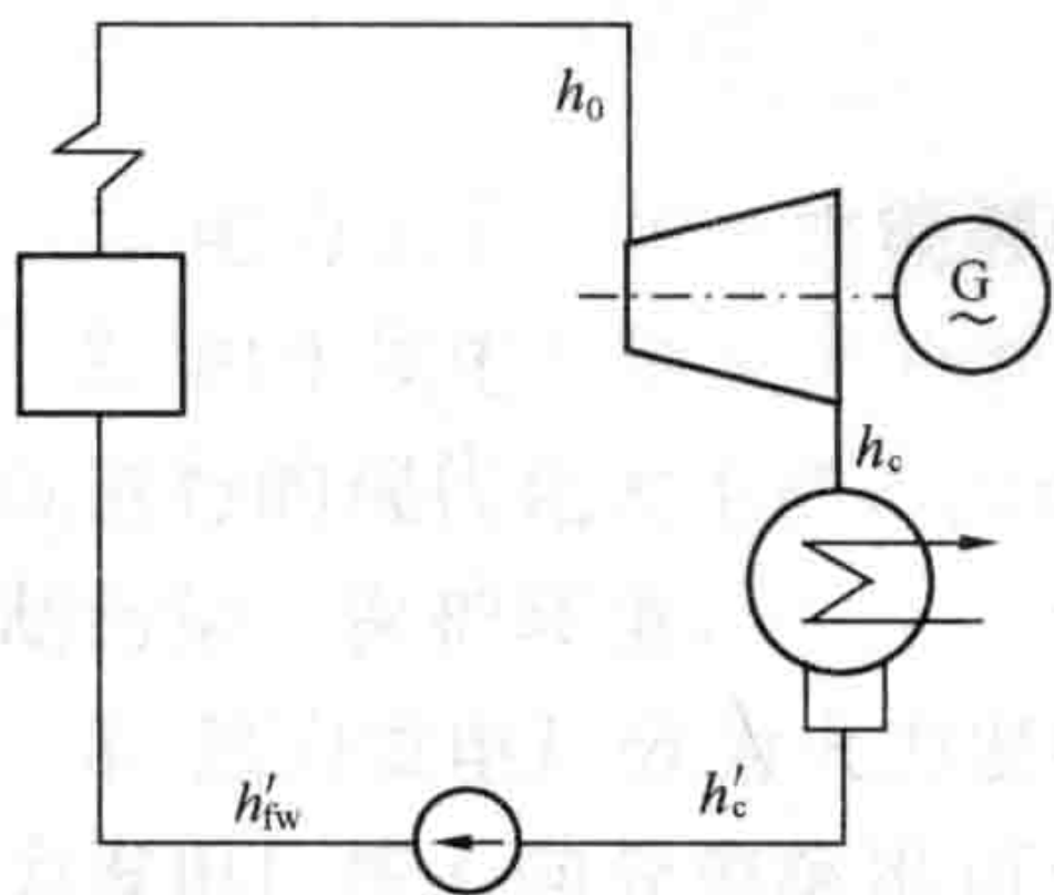
图 1-1 朗肯循环的热力系统
