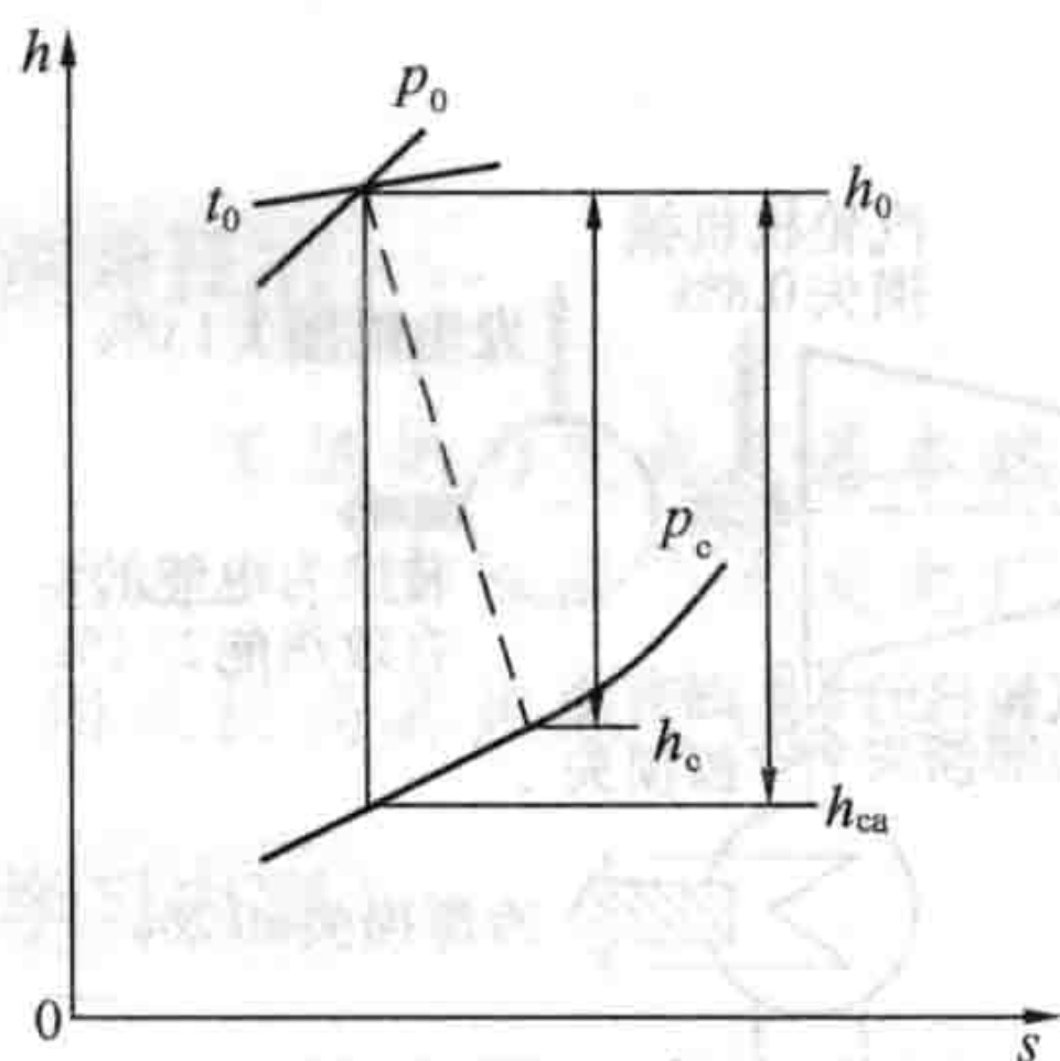
图 1-3 蒸汽在汽轮机中的焓降
