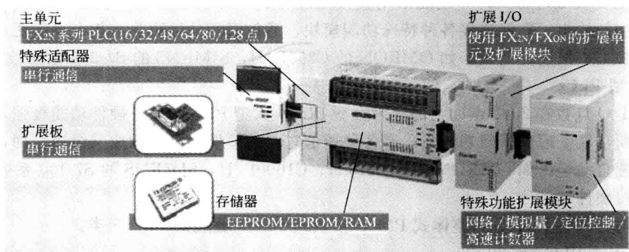
图 1-3 带扩展单元的 FX 2N 系列 PLC 的外形图
