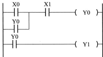
图 1-6 梯形图
