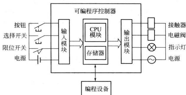
图 1-4 PLC 控制系统结构框图
