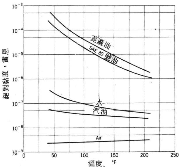
圖 10-2 各種常用流體之黏度比較
