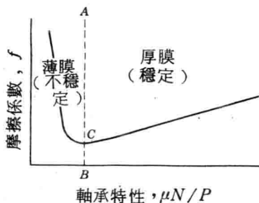
圖 10-4 摩擦係數與 \mu N/P 之變化
