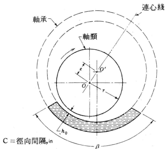
圖 10-6 頸軸承之術語
