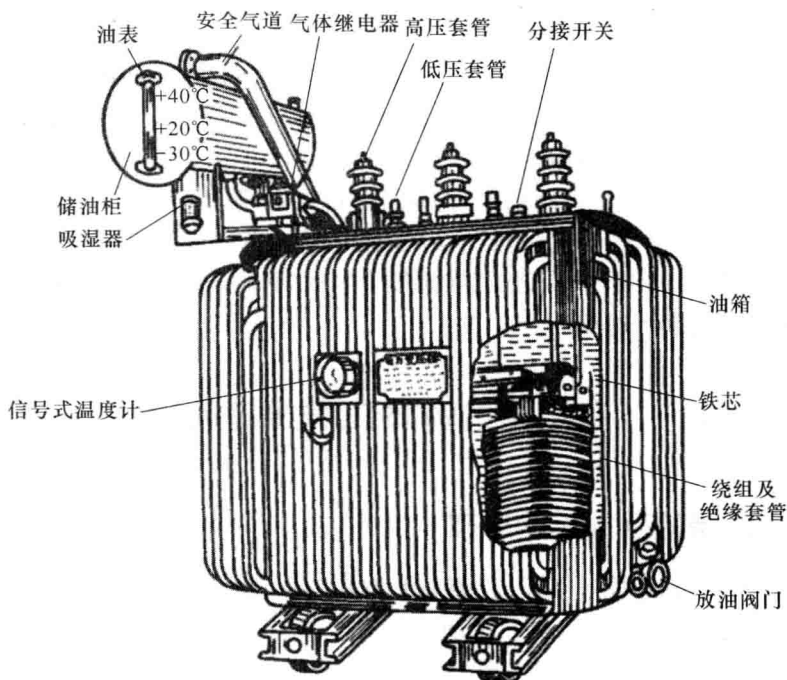
图 1.2 油浸式电力变压器
