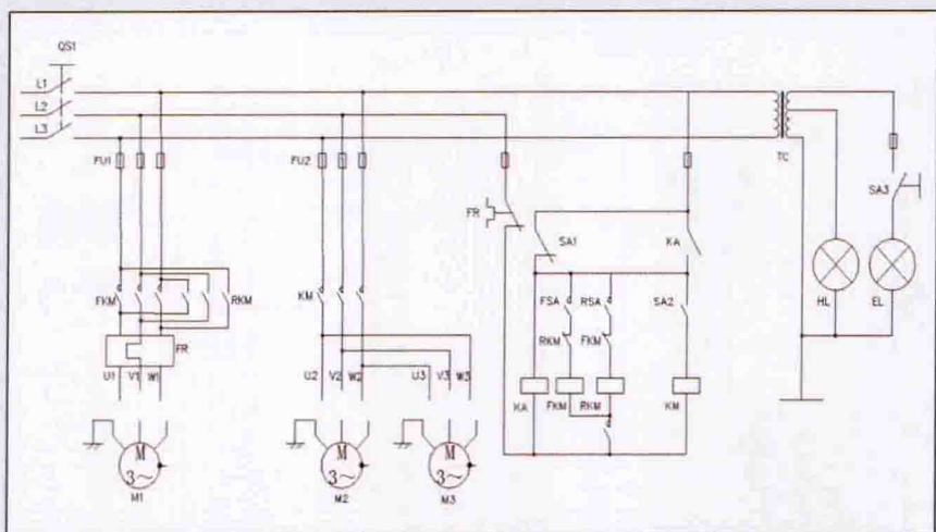
■ 车床电气图
