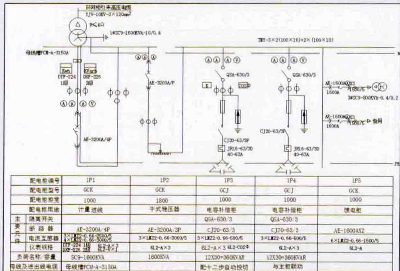
■ 工厂低压系统图
