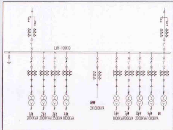
■ 变电工程图
