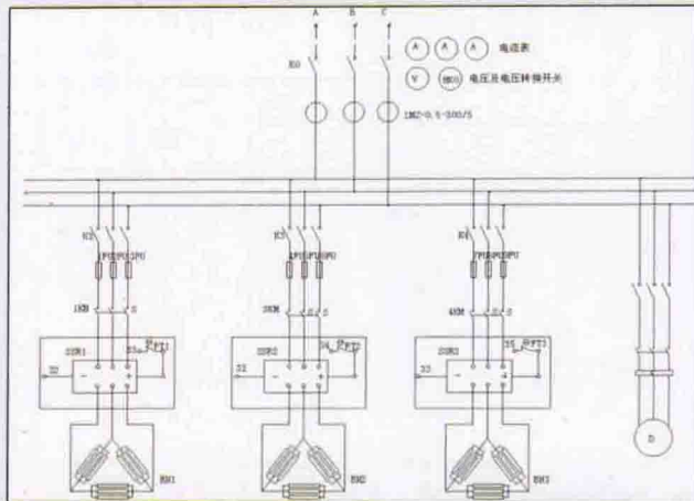
■ 烘烤车间电气控制图
