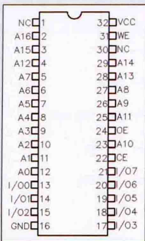
■ 单片机引脚图
