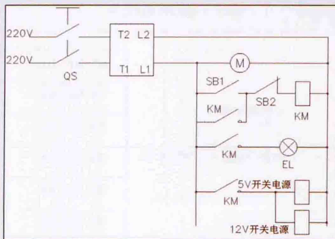
■ 电机驱动控制电路图
