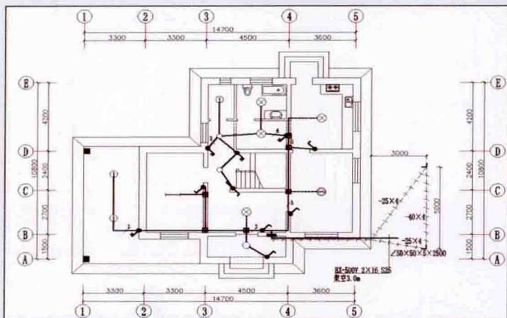
■ 一层照明平面图
