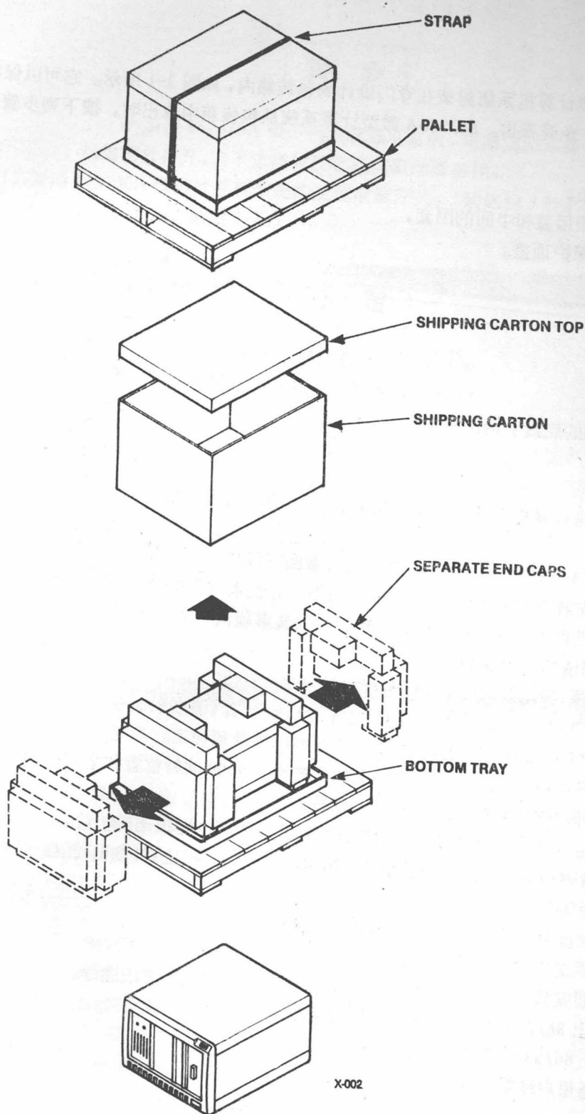
图 2-1 开箱图
