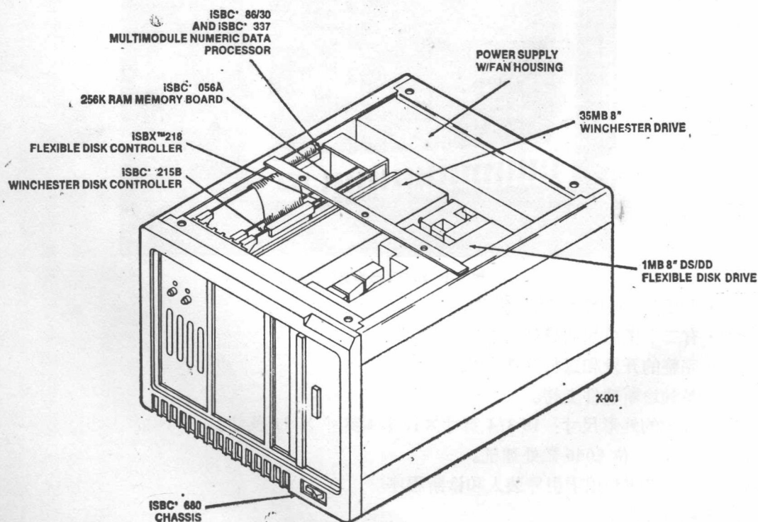
图 1-2 86/330内部位置图
