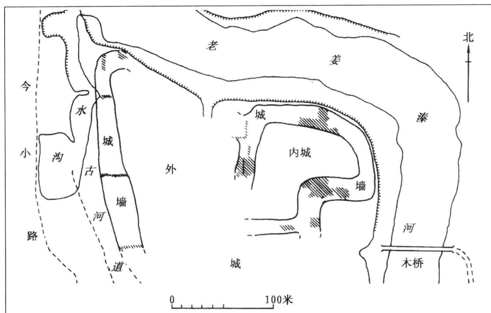
图1-3 天目山遗址城墙平面
