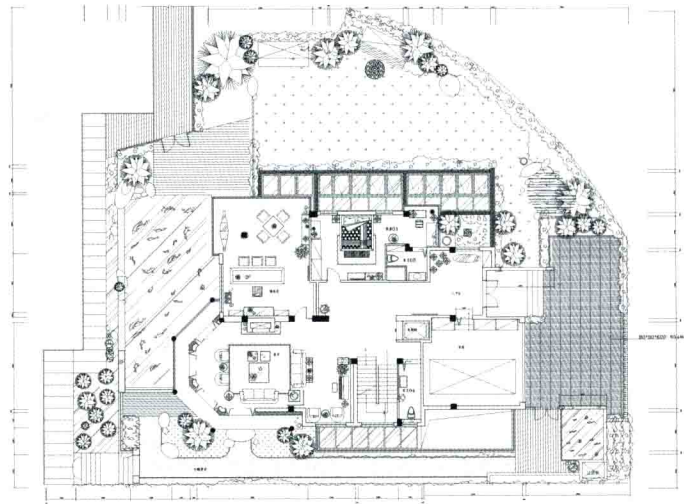
一层平面图
