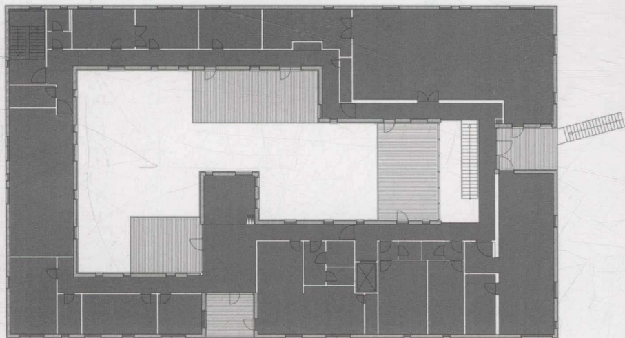
二层建筑平面图
