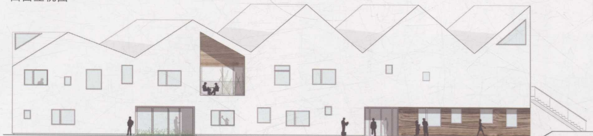
东面立视图
