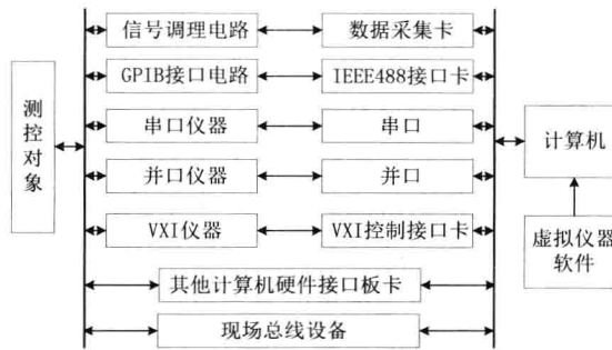
图 1-2 虚拟仪器结构框图
