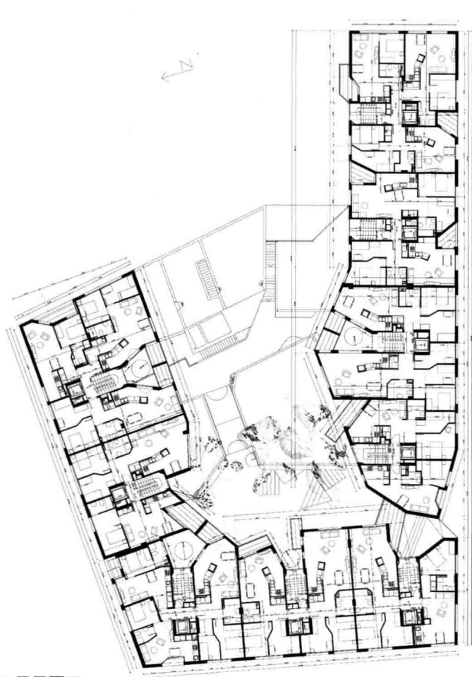
二层平面图
