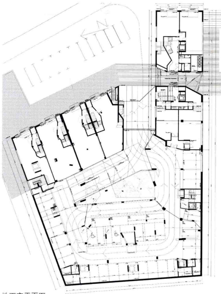
地下室平面图
