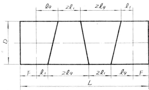
管子下料图
