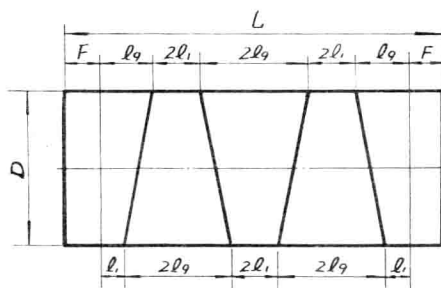
管子下料图
