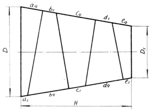
管子下料图
