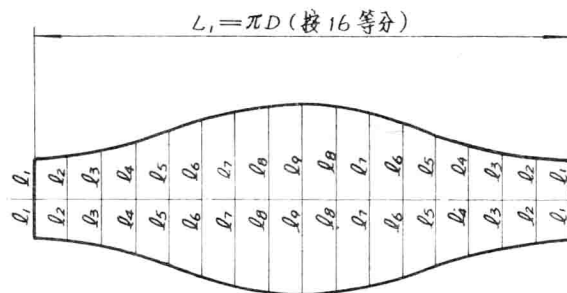
断节下料样板展开图
