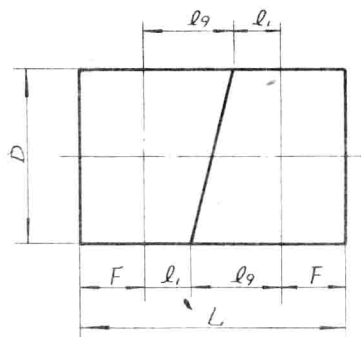
管子下料图
