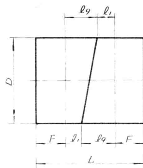
管子下料图
