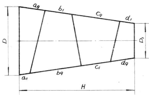
管子下料图
