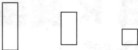
图 1-1 阳线的形态
