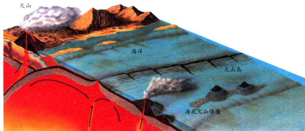
地壳及地幔示意图
