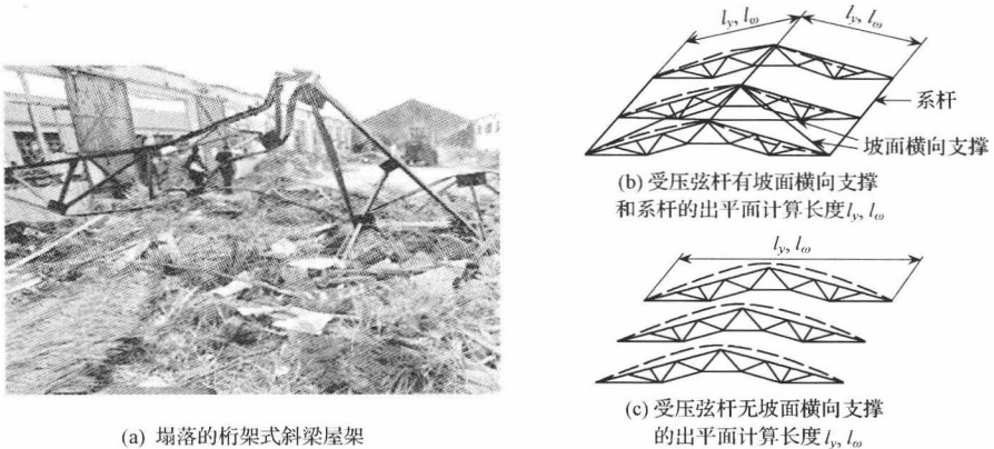
图 1 廊坊钢屋架塌落
