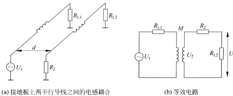
图 2-6 接地板上两平行导线之间的电感耦合及其等效电路
