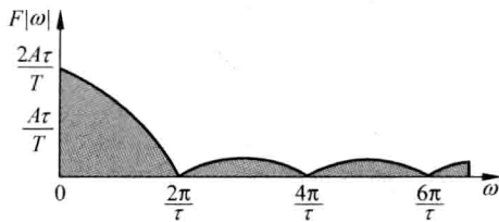
图 2-2 非周期性方波信号的频谱
