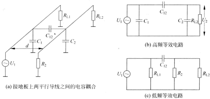
图 2-5 接地板上两平行导线之间的电容耦合及其等效电路
