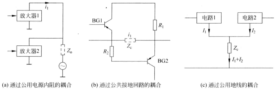
图 2-4 电阻性耦合
