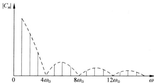
图 2-1 周期性方波信号的频谱
