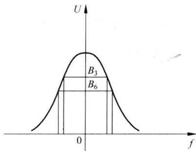
图 2-3 6dB 带宽和 3dB 带宽
