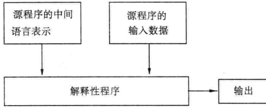
图 1.1 一个概念化的解释性程序
