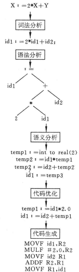
图 1.5 一个语句的编译过程
