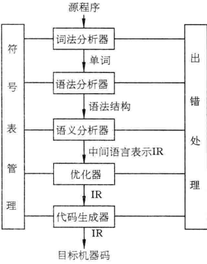
图 1.2 语法制导的编译程序的基本结构
