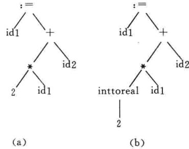
图 1.4 语义分析中插入一个从整到实的转换
