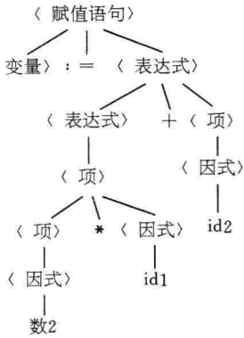
图 1.3 x := 2 * X + Y 的分析树
