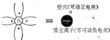
图 14-6 杂质半导体中的受主原子
