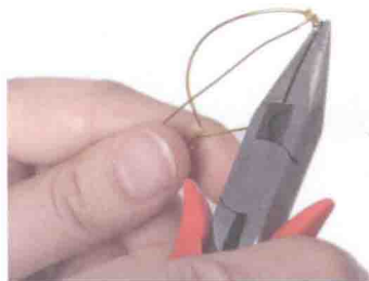
5. 再用尖嘴钳把另一头也拧紧。
