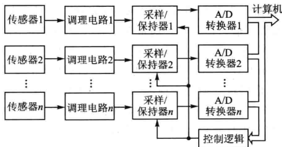
图 2-1-3 分散采集式模拟输入通道结构
