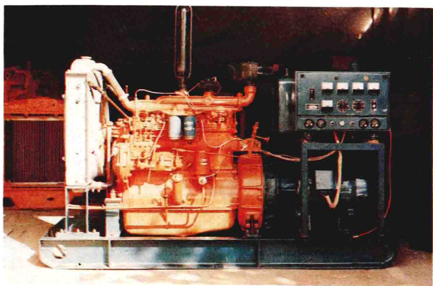
河北省新河发电设备厂生产的发电机
