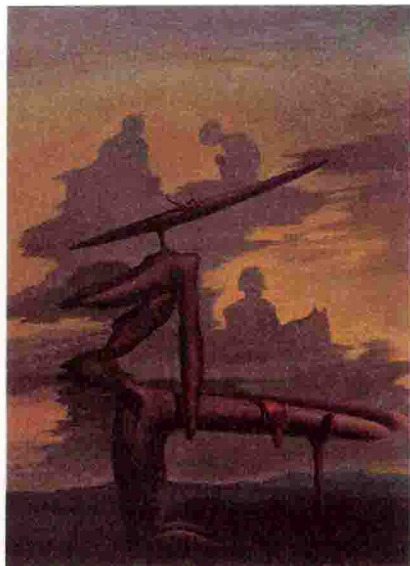
米勒光谱 (1934)
