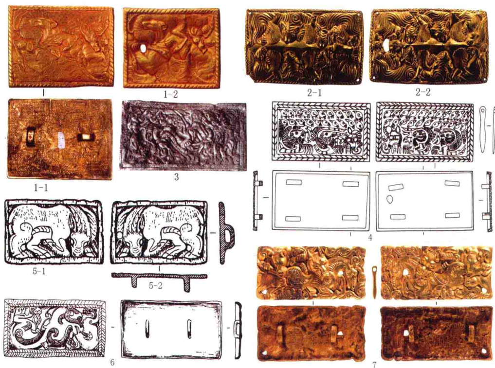
图版五 西汉墓葬出土的Aa型长方形腰饰牌
