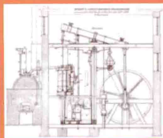
瓦特和他的蒸汽机专利图（1787年）
