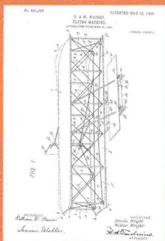
莱特兄弟和他们的飞机专利图（1906年）
