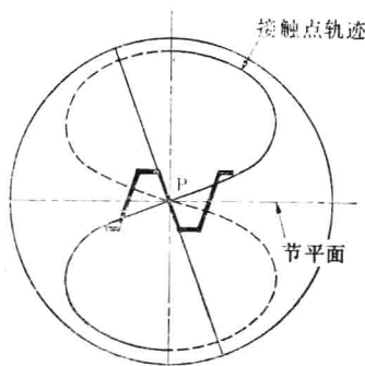
图 7-9 8 字齿形
