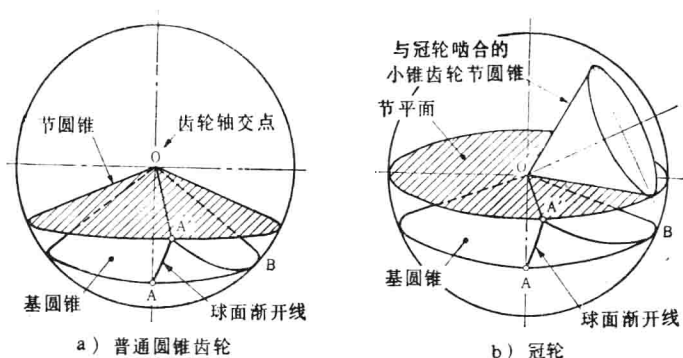
图 7-8 球面渐开线
