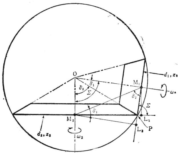
图 7-7 圆锥齿轮的节圆锥
