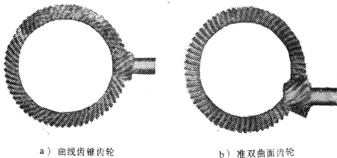
图 7-4 曲线齿锥齿轮与准双曲面齿轮
