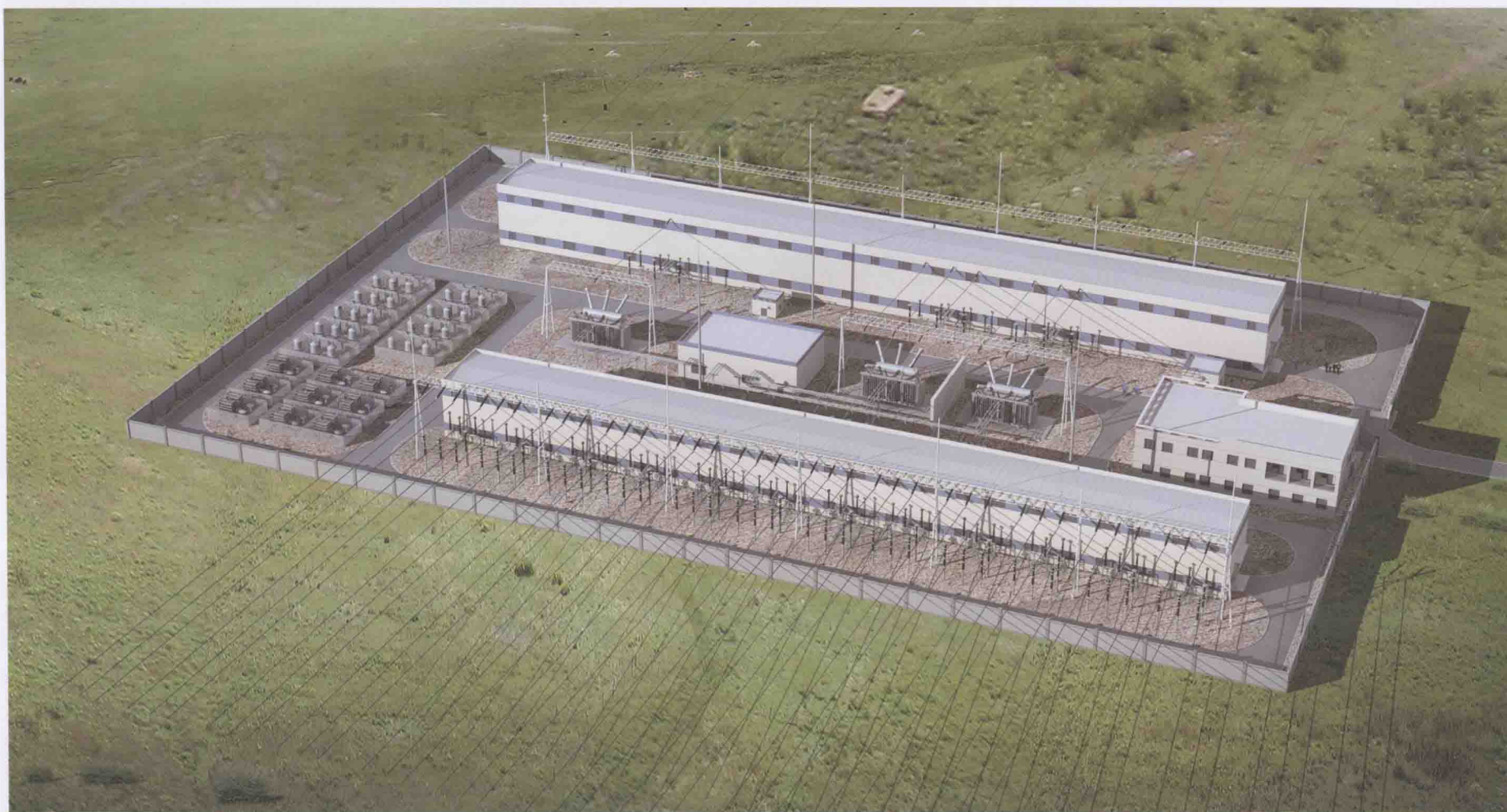
220kV变电站方案B—1鸟瞰图
