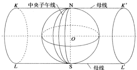
图 1-9 高斯平面直角坐标的投影
