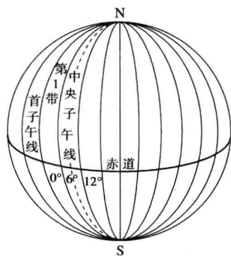
图1-7 高斯投影分带示意图
