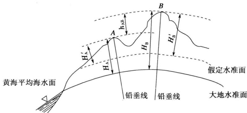
图 1-4 地面点的高程
