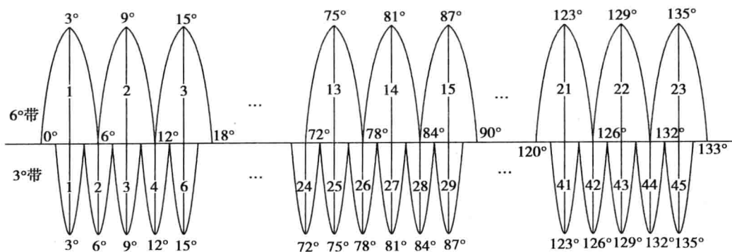
图 1-8 6°带、3°带中央子午线及带号
