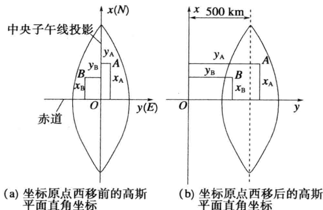
图 1-10 高斯平面直角坐标
