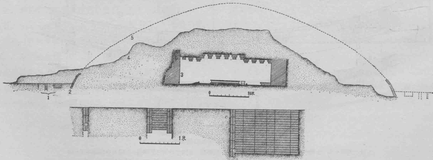
图六 王建墓陵台纵剖面图
