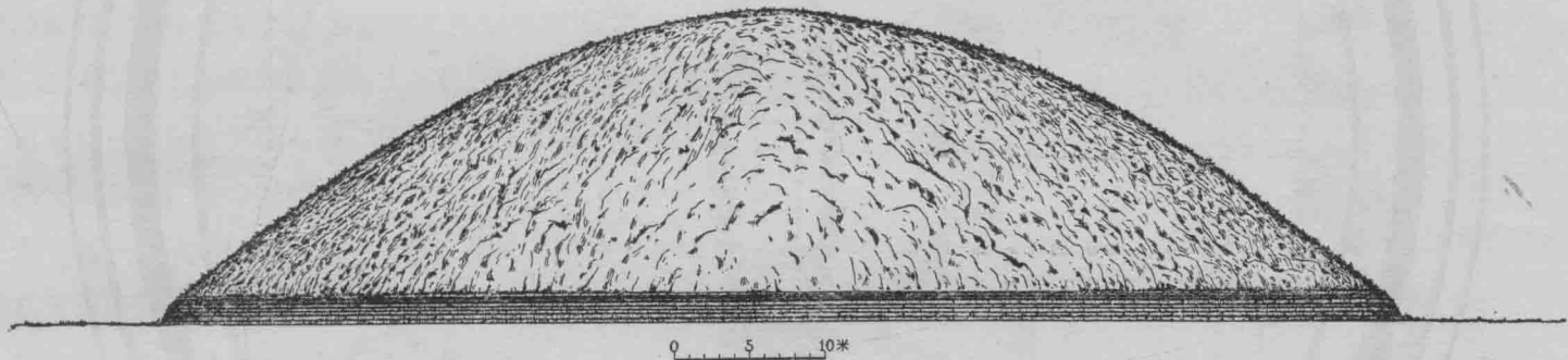
图三 王建墓陵台外形复原示意图
