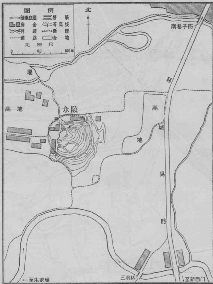
图二 王建墓陵台实测图(1942 年測繪)
