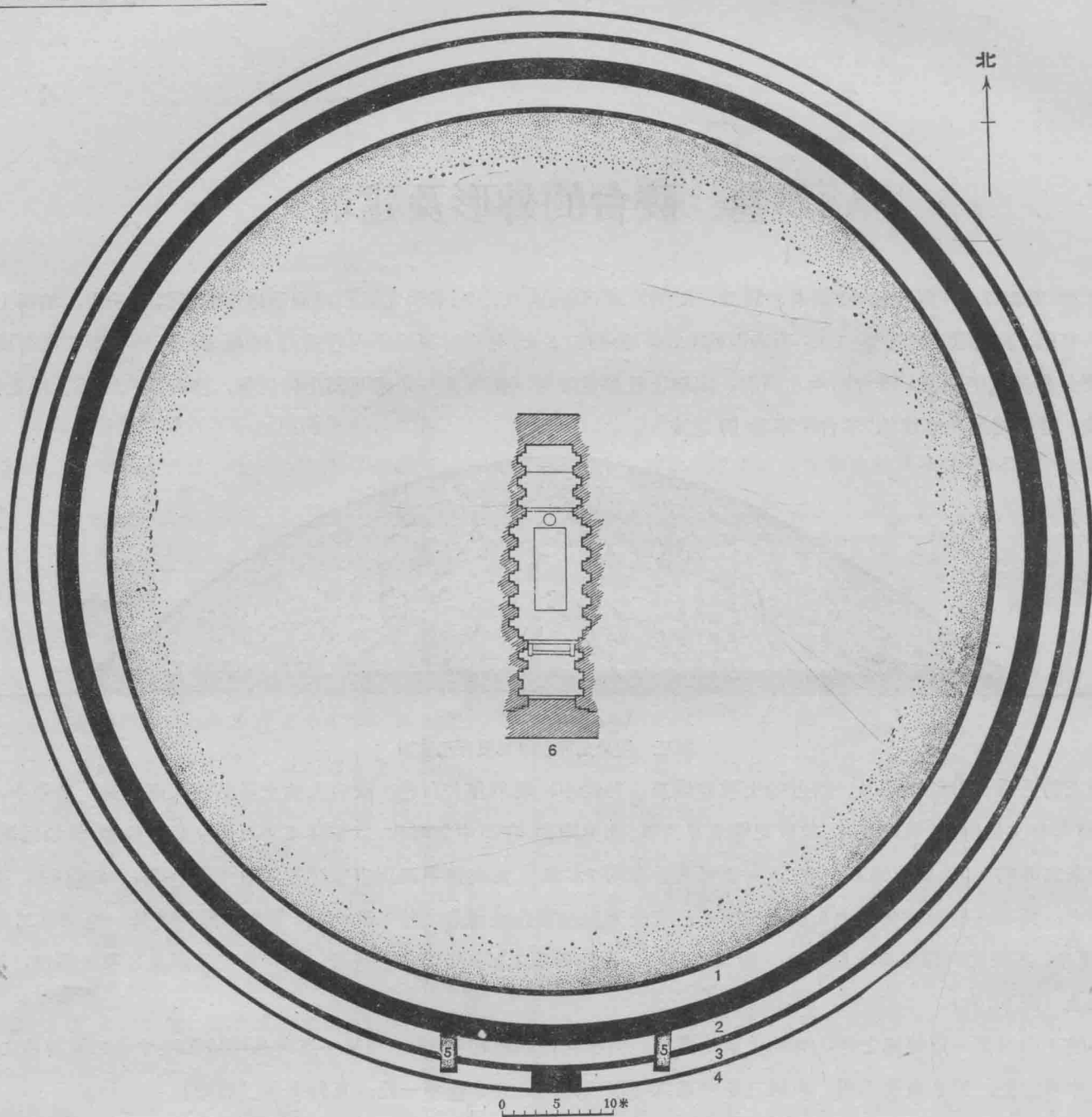
图五 王建墓陵台平面图
