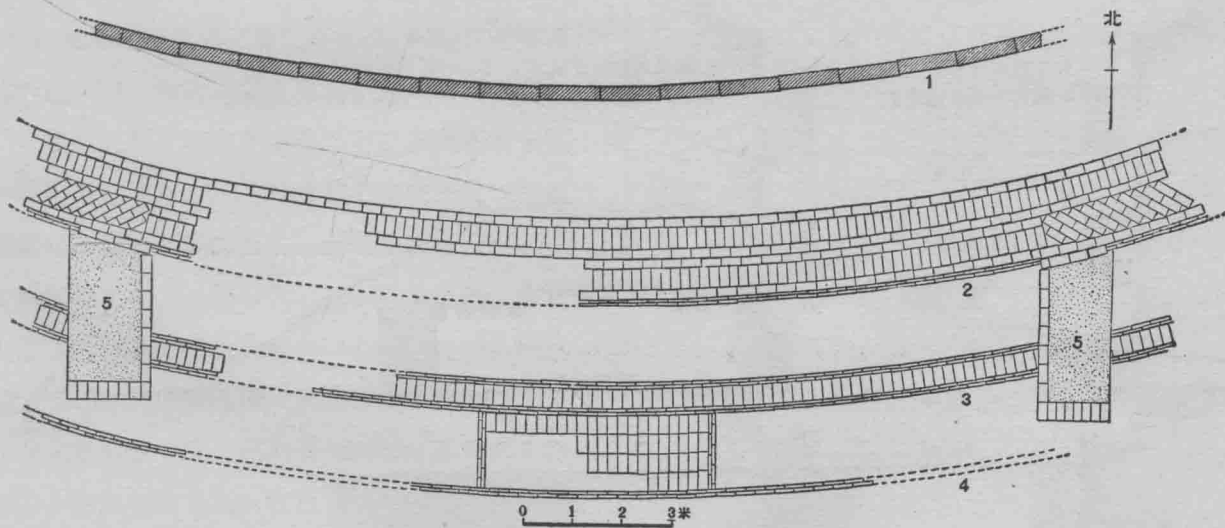
图四 王建墓陵台南面基脚結構平面图
