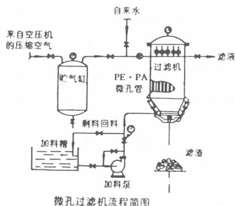
微孔过滤机流程简图
