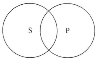
图 1—3 交叉关系欧拉图
