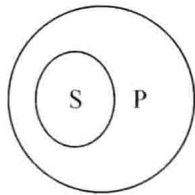
图 1—2 真包含关系与真包含于关系欧拉图
