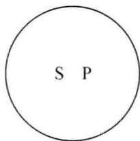
图 1—1 全同关系欧拉图
