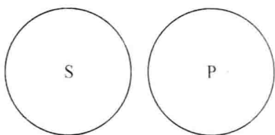
图 1—4 全异关系欧拉图
