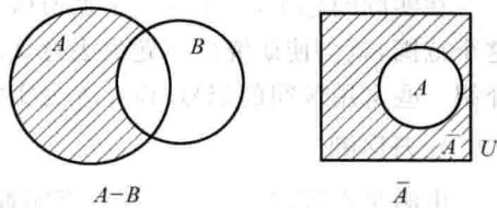
图 1-2 差集与补集
