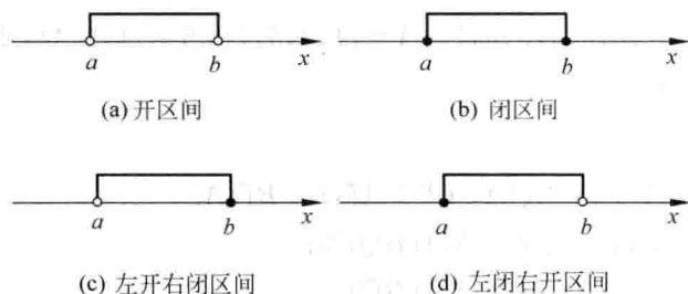
图 1-3 区间示意图
