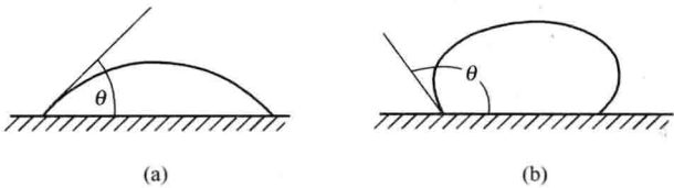
图 1-1 材料的润湿性示意图
