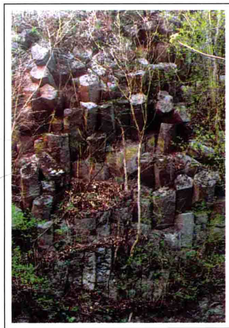
玄武岩柱体
