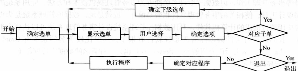
图 1-1 管理信息系统的系统控制方法示意图
